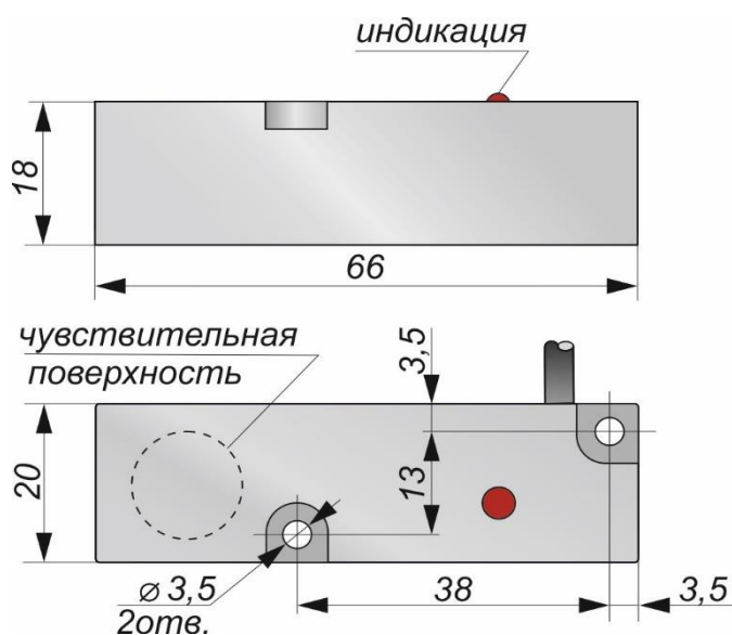
Габаритный чертеж
